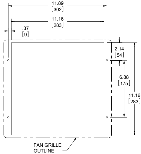
CUTOUT DIMENSIONS
