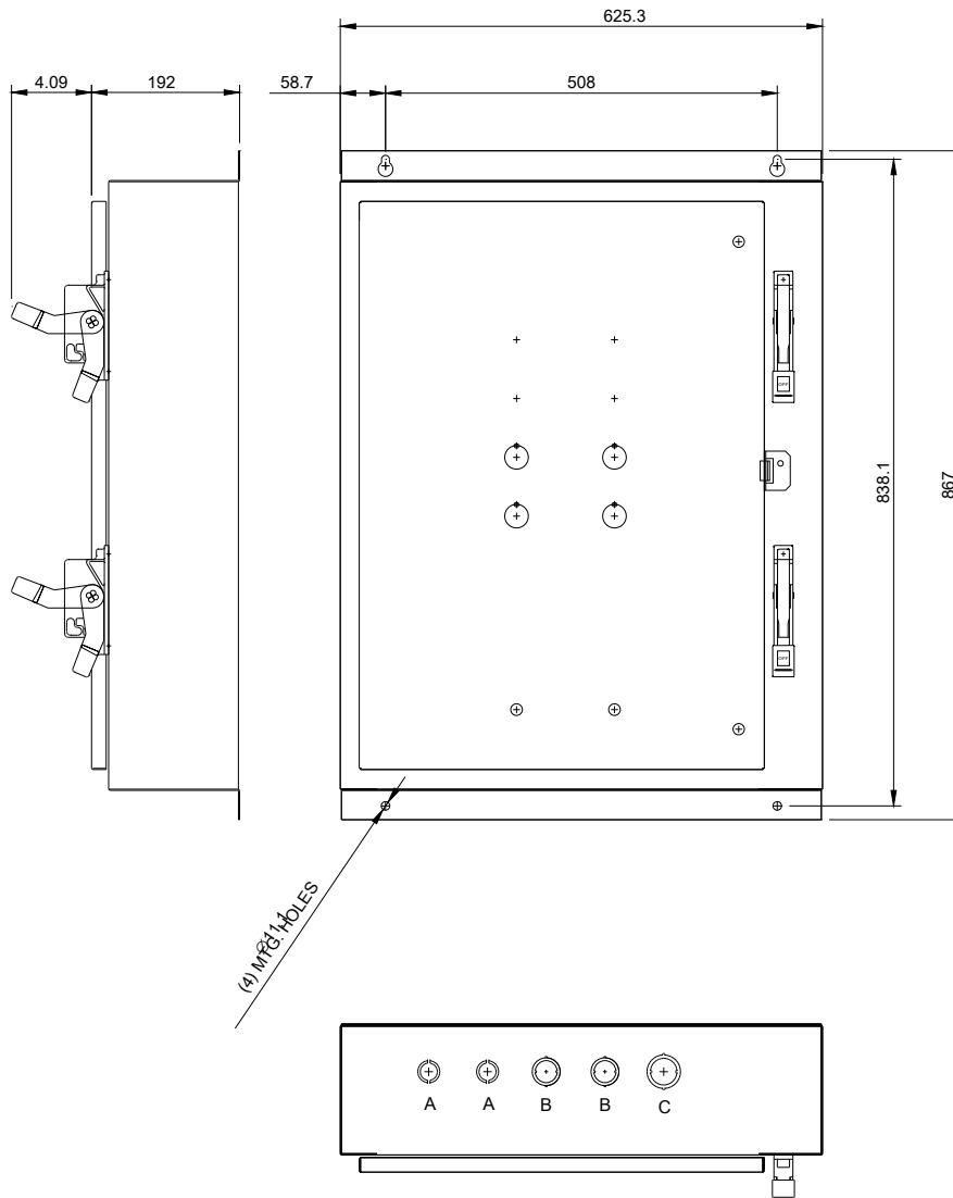
\\CONDUIT TYP. TOP AND BOTTOM
