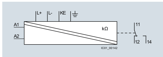
3UG4582
