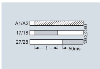
YΔ 3RP2005-.B Wye-delta function
