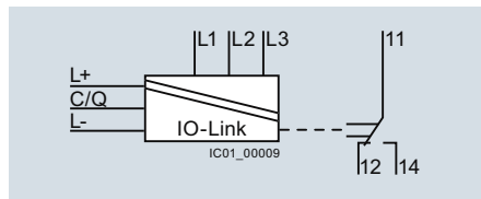
3UG4815
