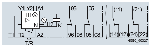
3RN1013-...1 (bistable)
