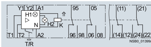
3RN1012, 2 CO
