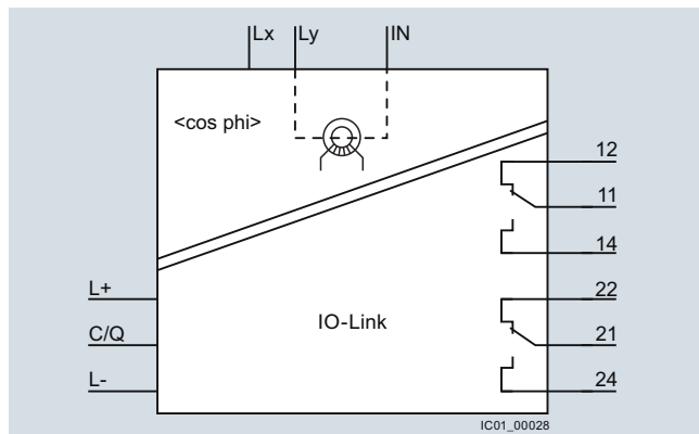
3UG4841
