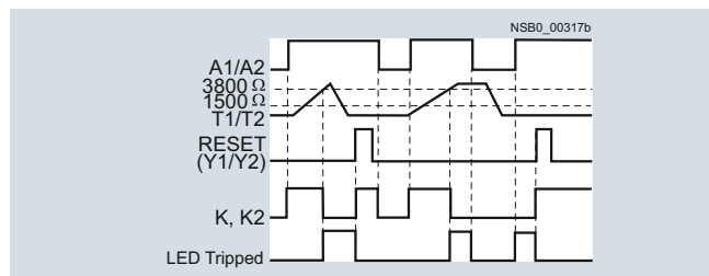
3RN1012/3RN1022/3RN1062 1)
