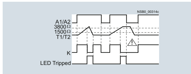
3RN1011 1)
