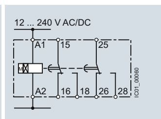
7PV1508-1BW30 ON-delay
