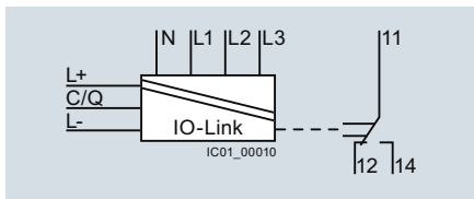
3UG4816
