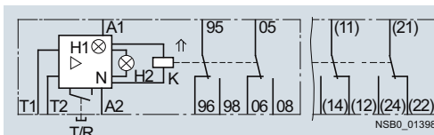
3RN1011, 2 CO
