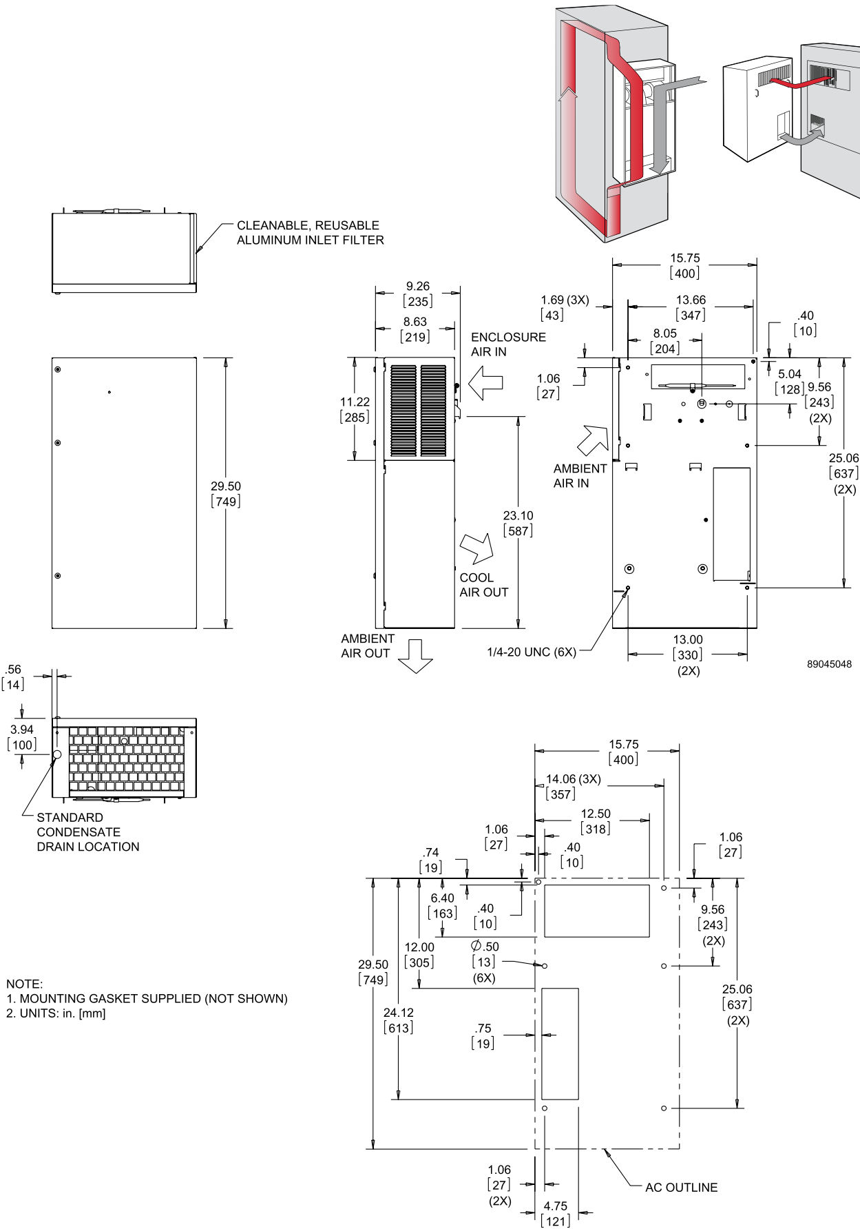
Cutout Dimensions
