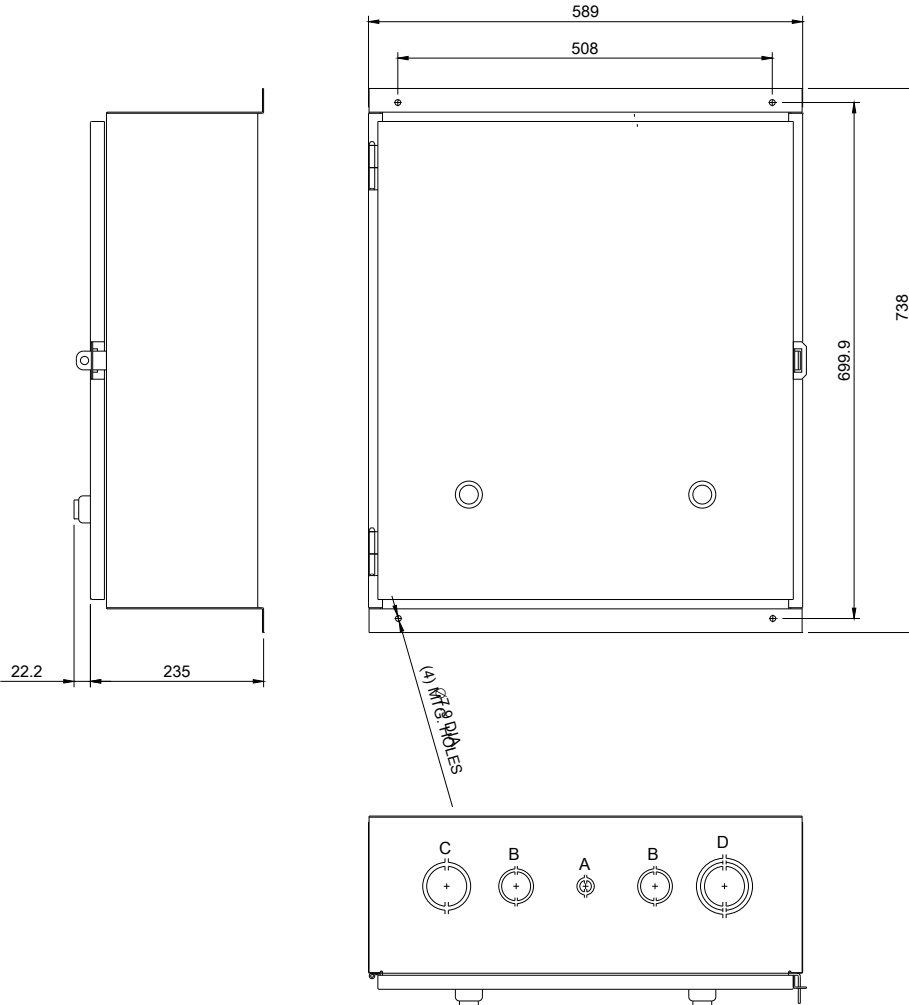
\\CONDUITS TYP. TOP & BOTTOM
