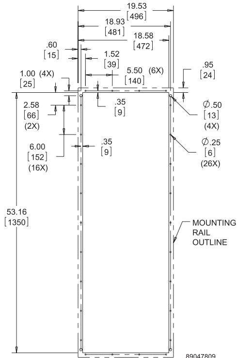
Cutout Dimensions
