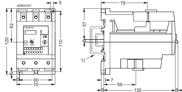
3RU11 46 --.D.
